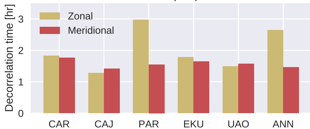
Data (FPI)
