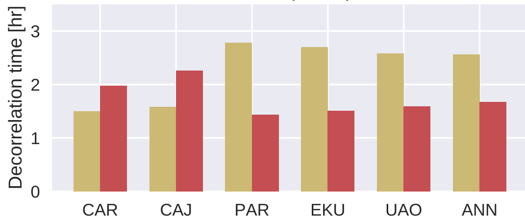
Model (GITM)
