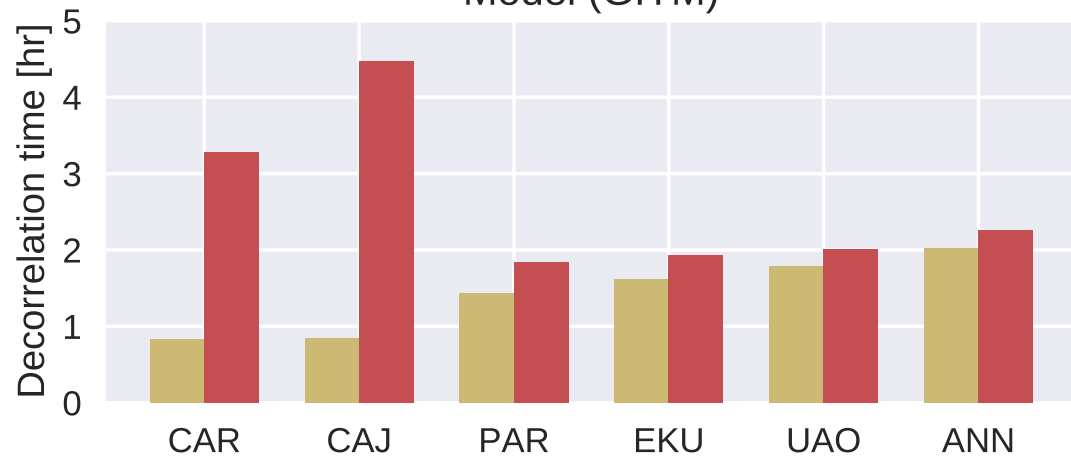
Model (GITM)
